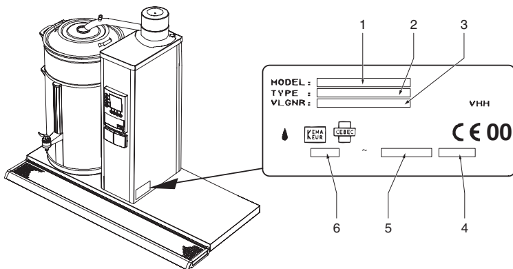
Fig. 1 Identificatieplaatje
