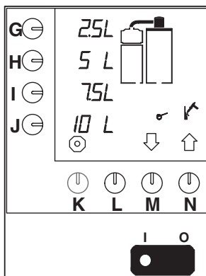
Fig. 3 Bedieningspaneel koffiezetstelsel
