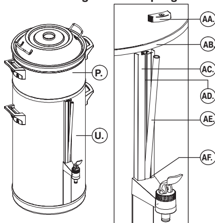
Fig. 8 Reinigen van het peilglas
