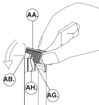
Fig. 9 Plaatsen en verwijderen peilglaskapje
