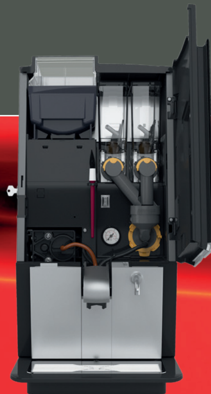
Esprecious 22 med delt bønnebeholder og 2 instantbeholdere
