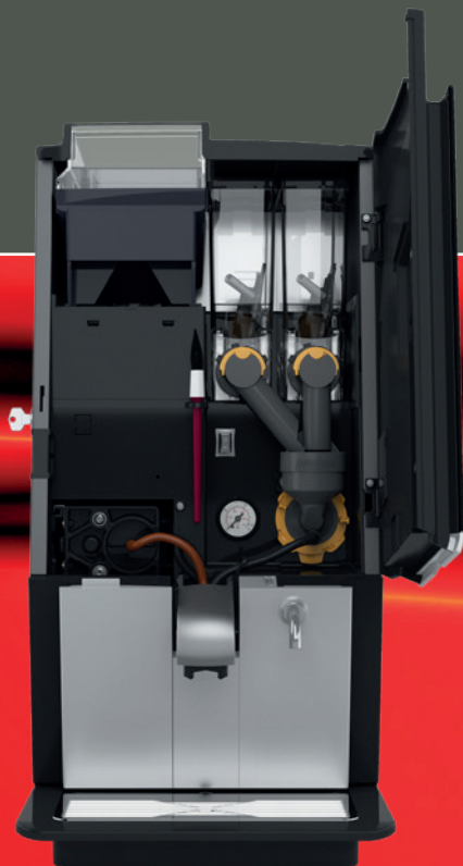
Esprecious 12 med 1 bønnebeholder og 2 instantbeholdere
