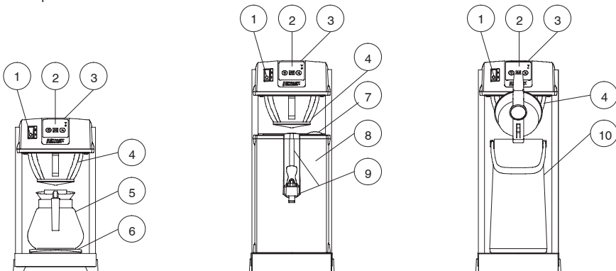
Fig. 1 Composants principaux des modules café
