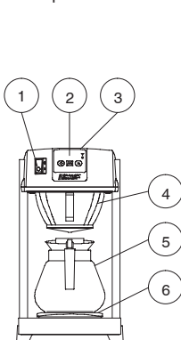
Fig. 1 Hoofdcomponenten koffie modules
